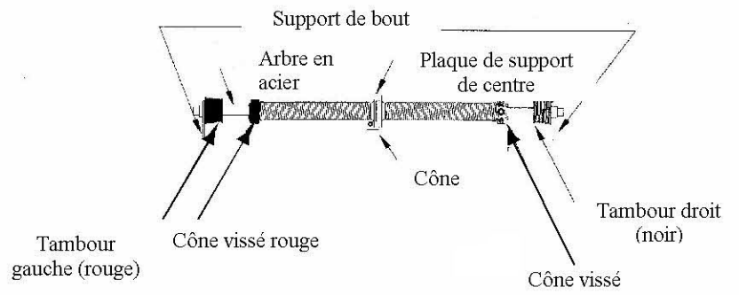
Ressort à torsion
