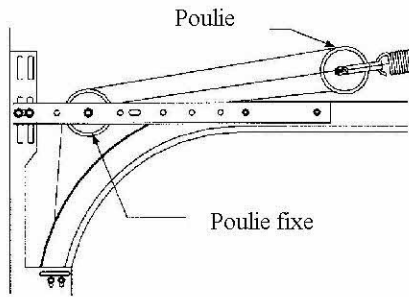
Ressort à extension
